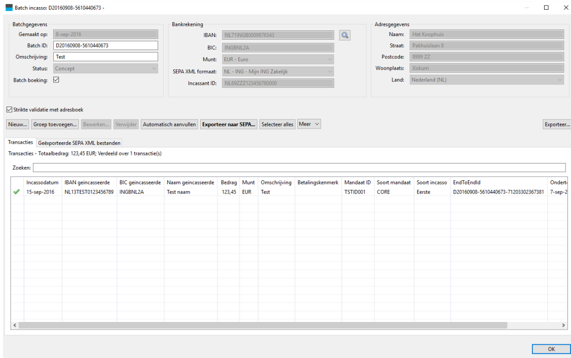
Figuur 4: Verzamelopdracht met een gevalideerde transactie
